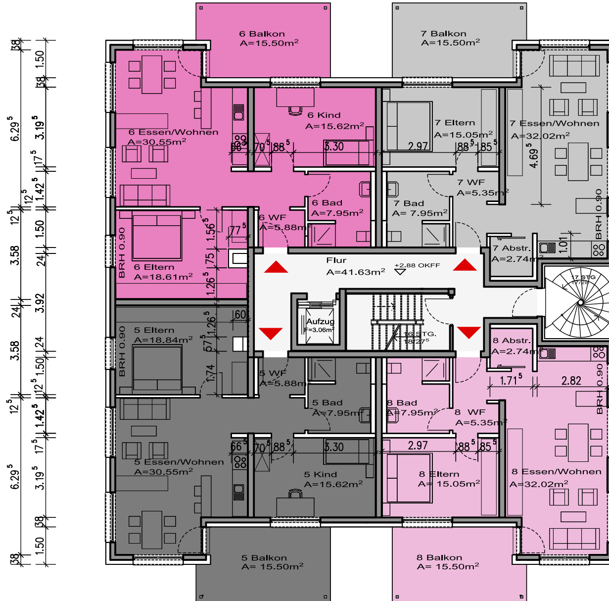
1.0G Haus V Wohnungen 5-8
